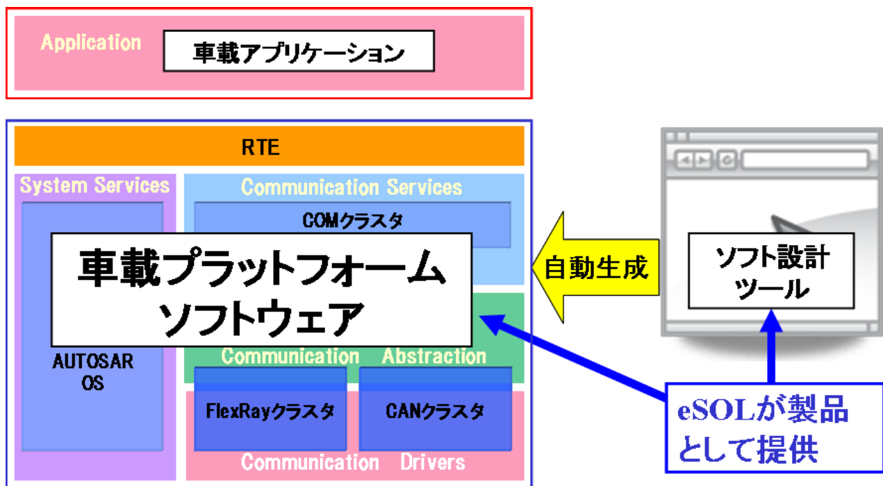
図1 車載プラットフォームソフトウェアとソフト設計ツール
